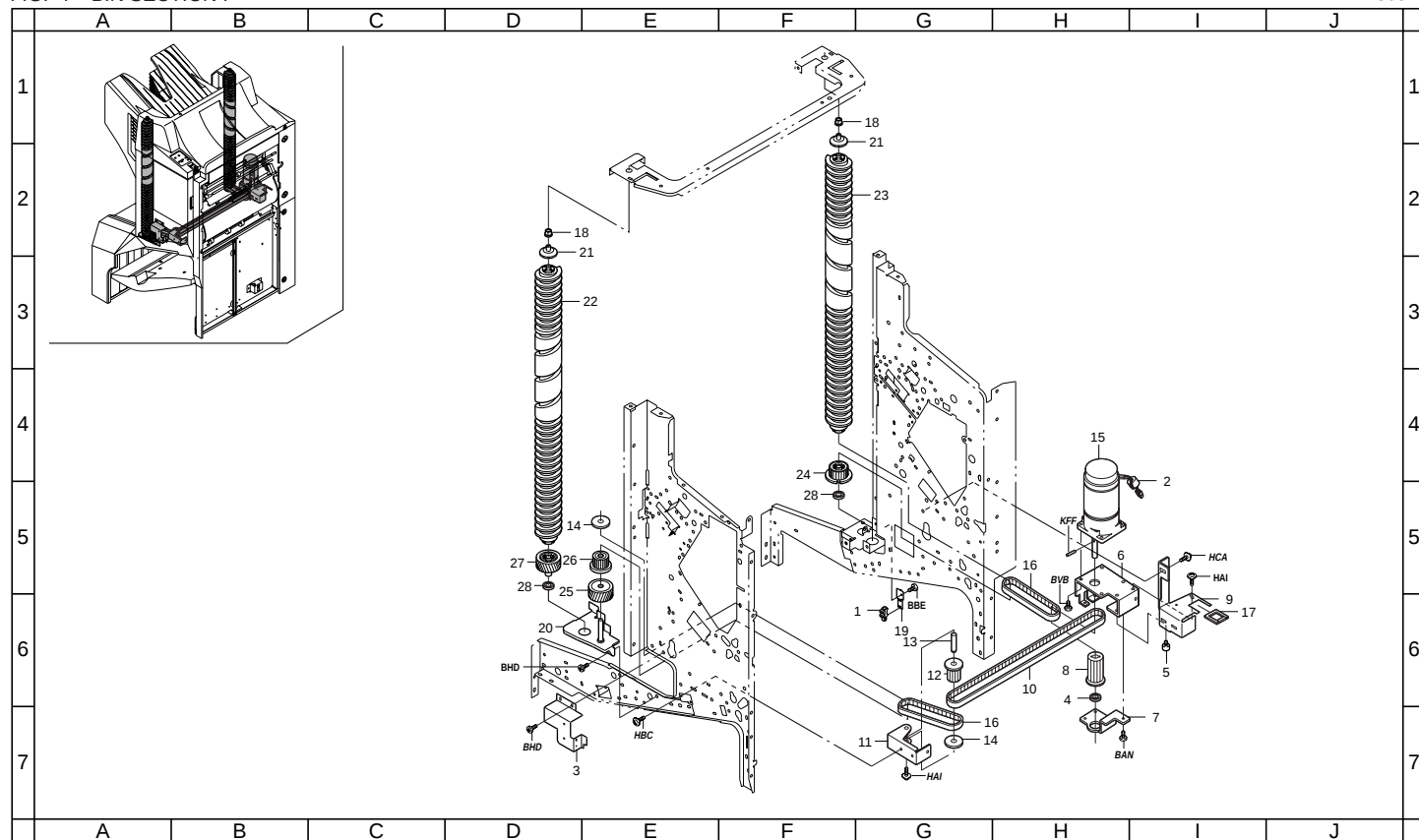
FIG. 4 BIN SECTION I
